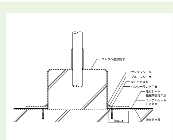
架台部 (ウレタン塗膜防水併用)
