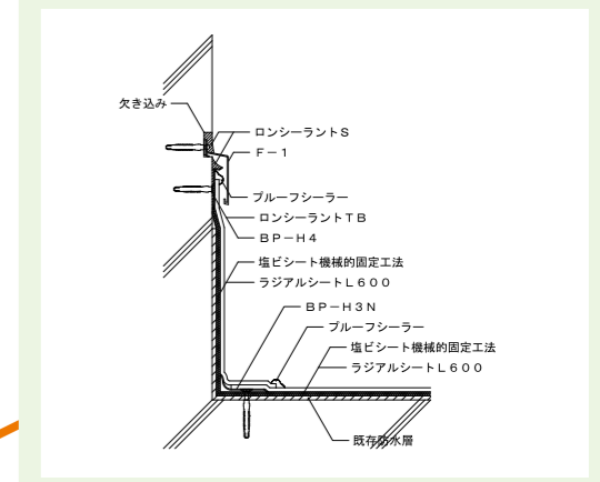
壁部
