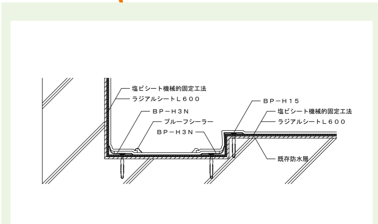
側溝部
