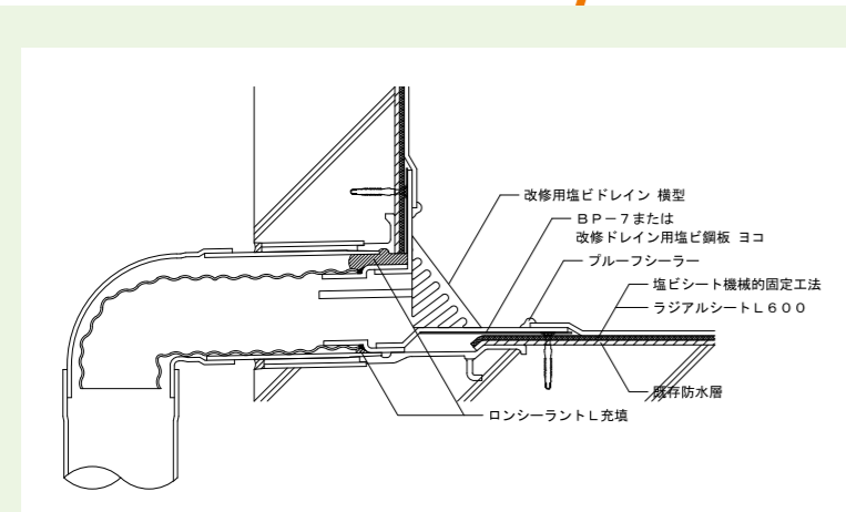
ドレイン部
