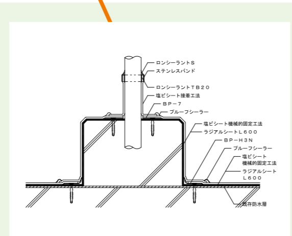
架台部 (シート巻き込み)
