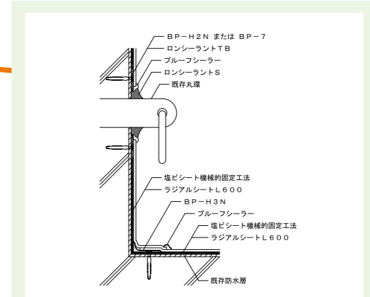
吊環部
