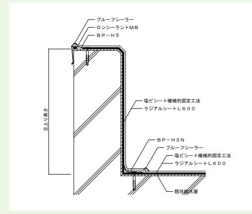
パラペット (あごなし)
