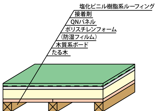
▲屋上防水断面詳細イメージ
